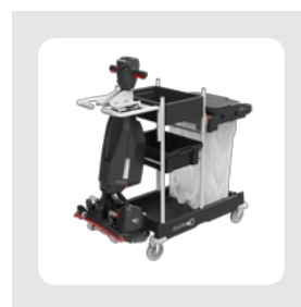
917016 Carro ServoMatic SM5 1120 x 580 x 1150 mm Contenedor de residuos: 120 l
